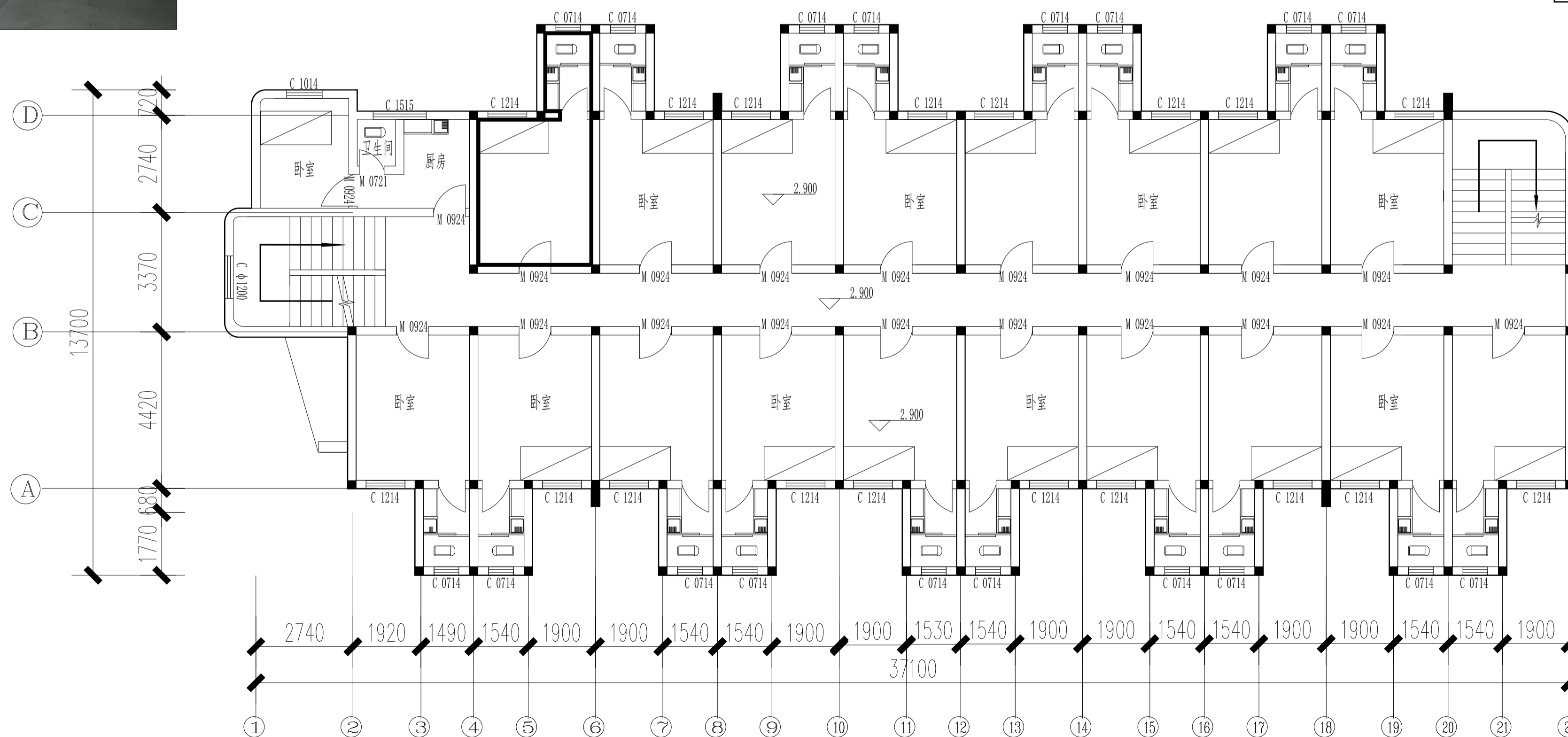
二~五标准层平面 (改造前)
