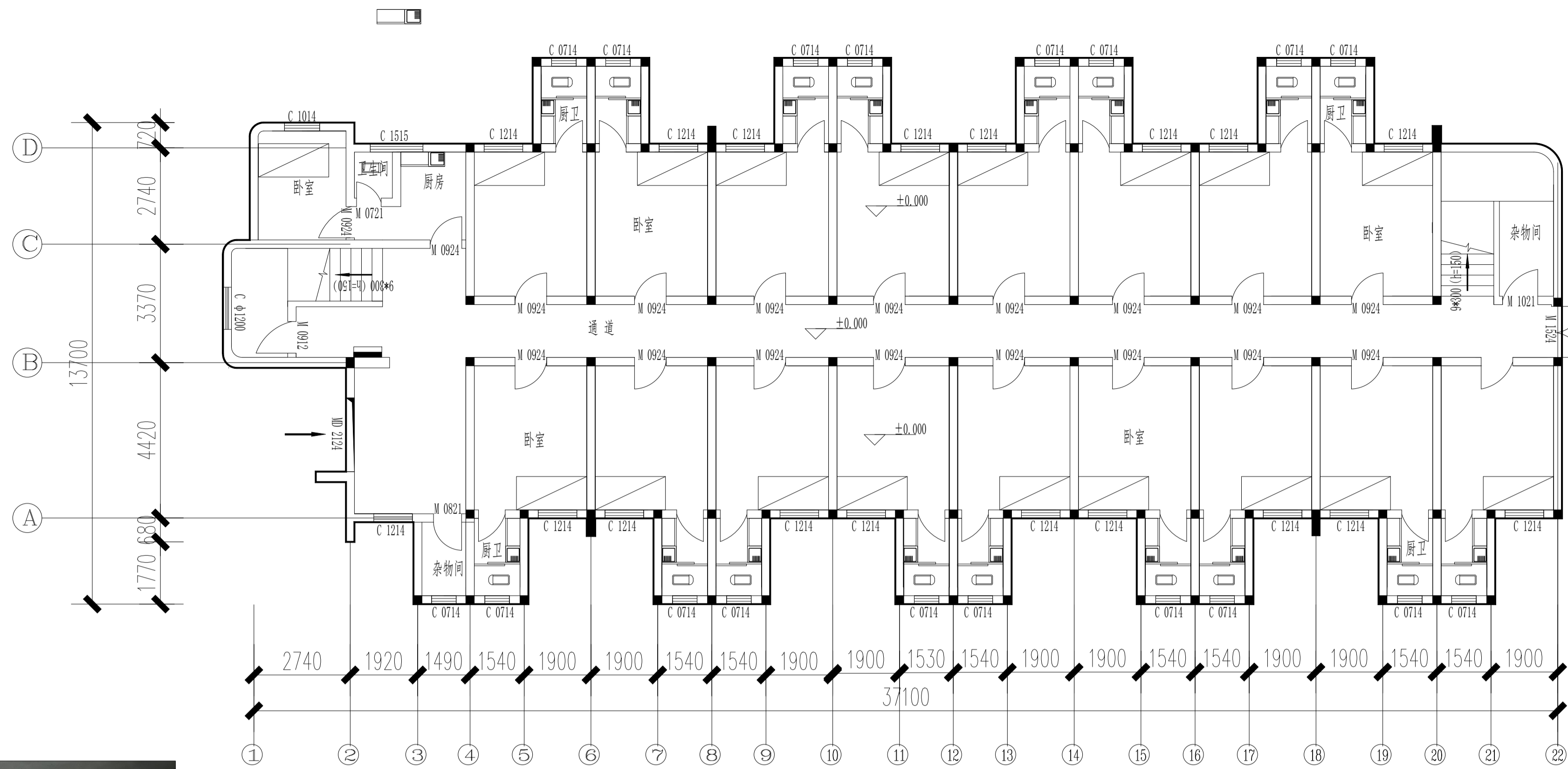
首层平面图 (改造前)
